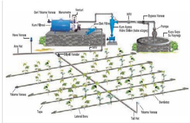
Şekil 17. Damla sulama elemanları.
